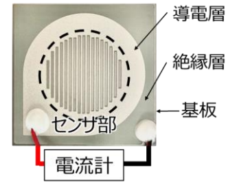
ACMセンサ外観
