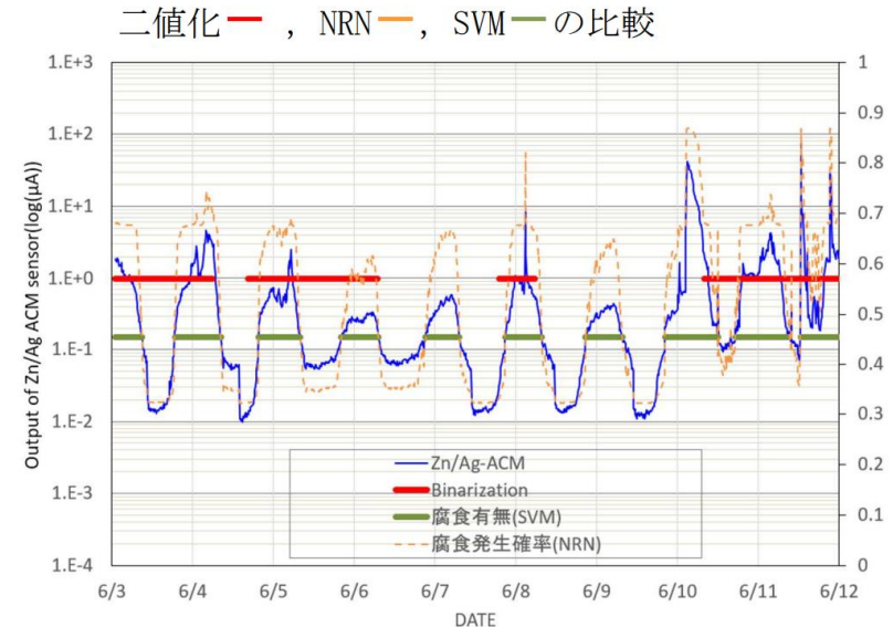
AI(人工知能)を使ったZnめっきの腐食解析
